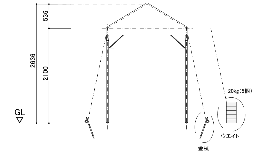
立面図 1/50
