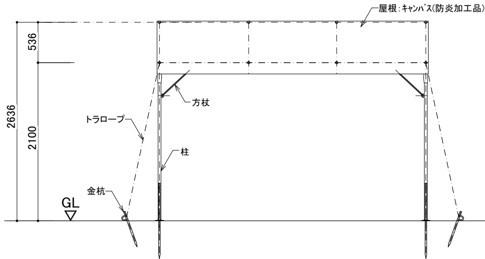
立面図 1/50
