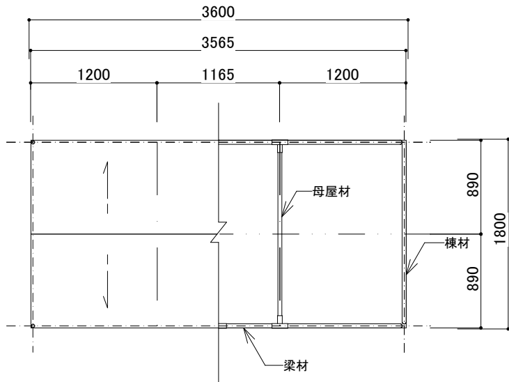
屋根・小屋伏図 1/50
