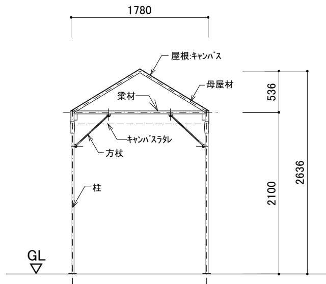
断面図 1/50
