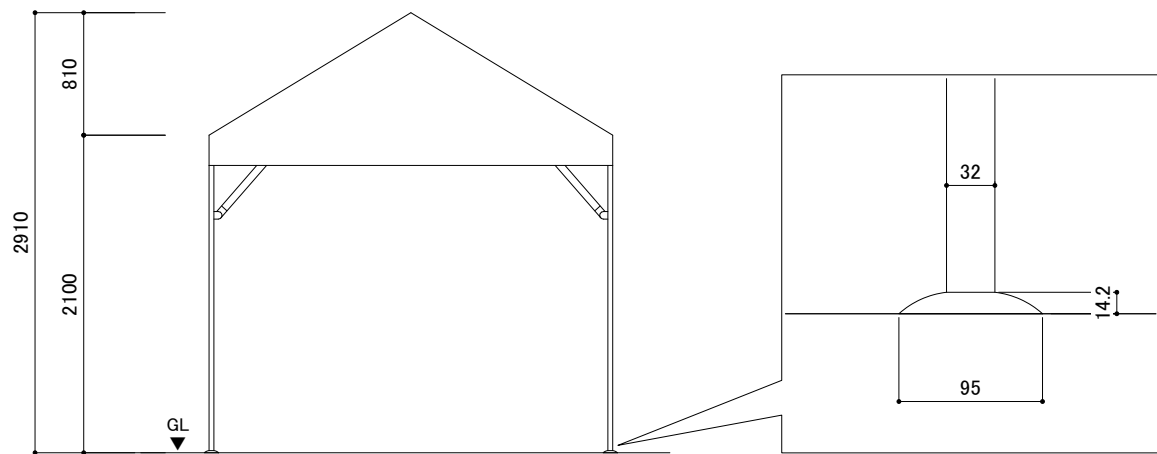
立面図
