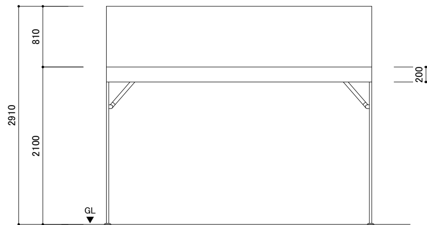
立面図
