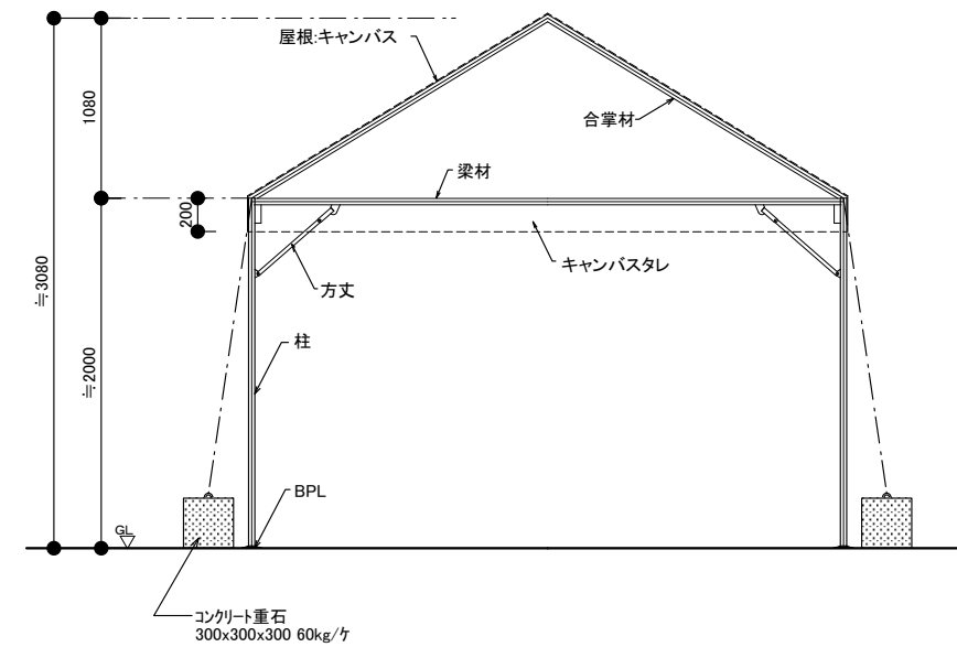
断面図 1/50
