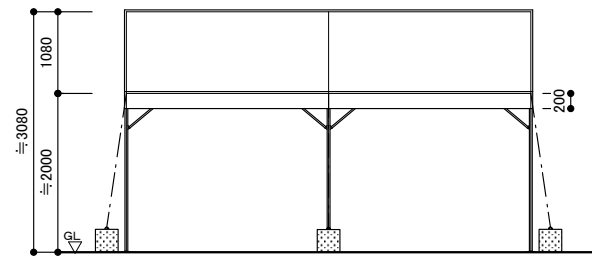
立面図 1/100
