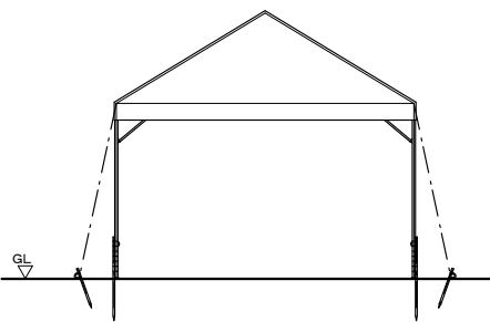
立面図 1/100
