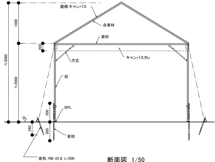
断面図 1/50
