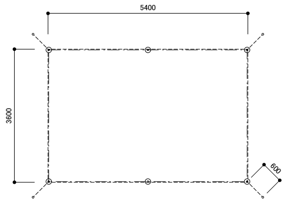
平面図 1/100
