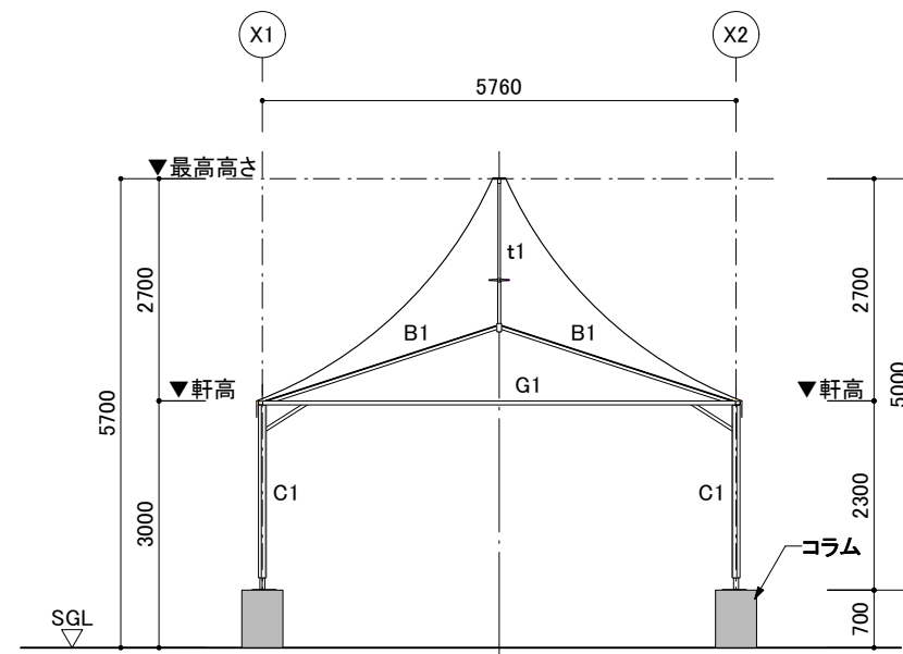
軸組図 S=1/100
