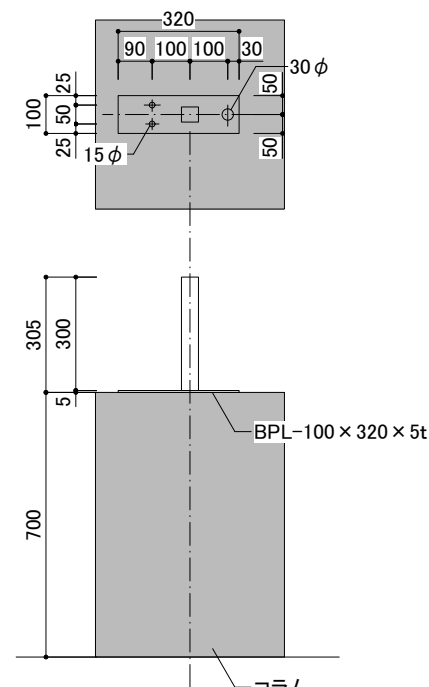
柱脚詳細図 S=1/10
