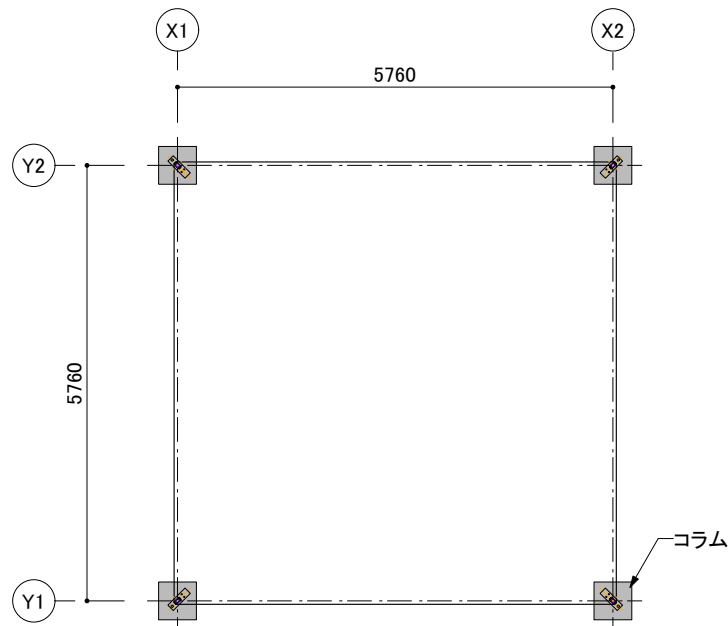
平面図 S=1/100
