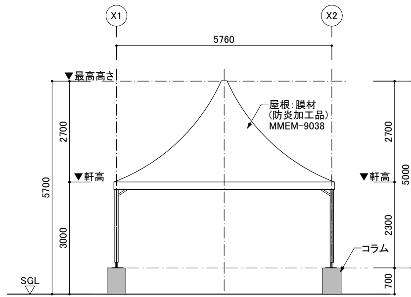
立面図 S=1/100
