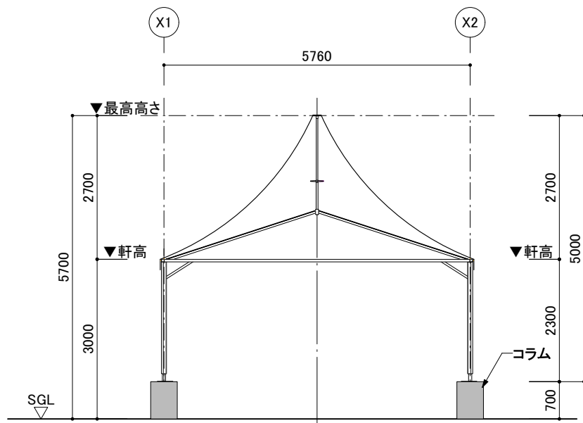
断面図 S=1/100
