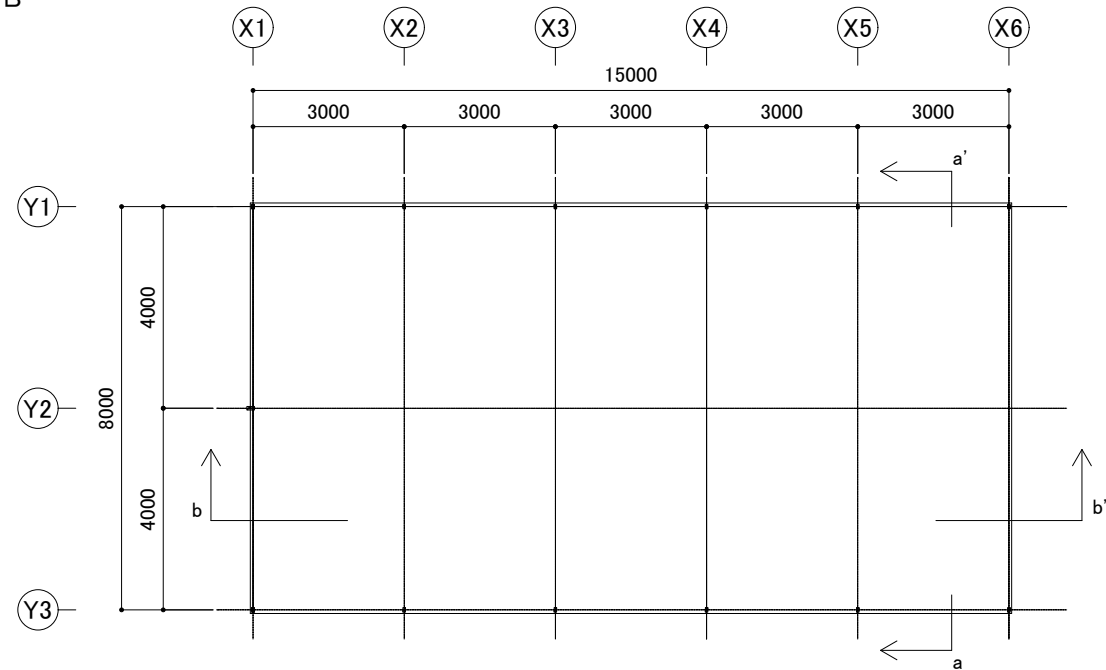
平面図 S=1/150
