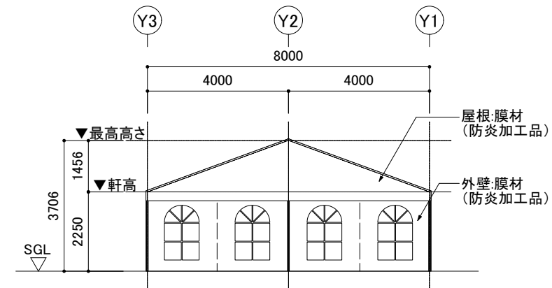
B立面図 S=1/150
