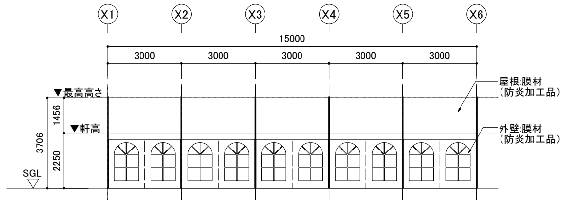
A立面図 S=1/150
