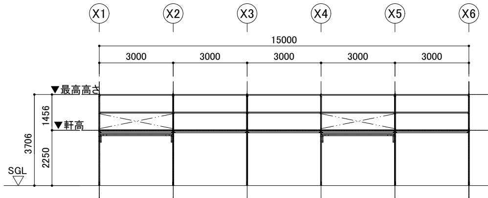
b-b'断面図 S=1/150
