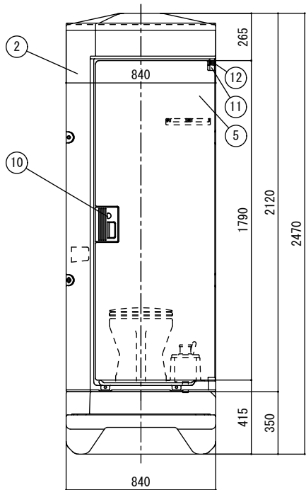
正面図
