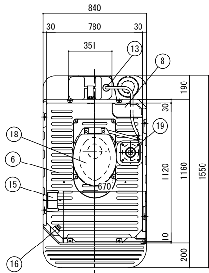
平面図
