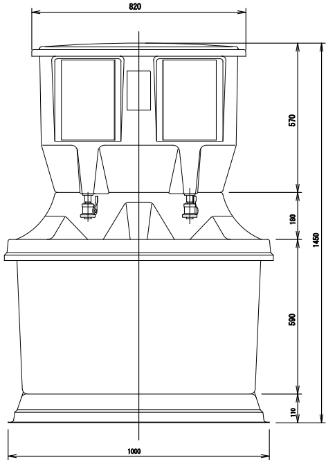
正面図 S=1/20
