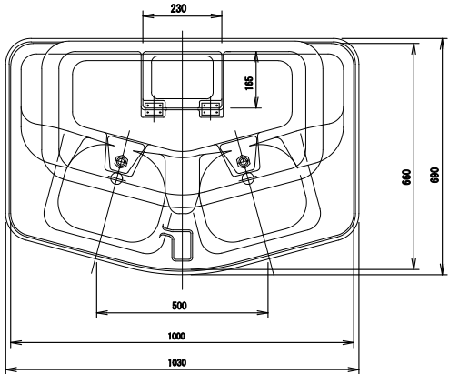
平面図 S=1/20
