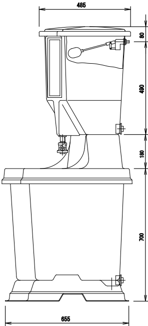
側面図 S=1/20
